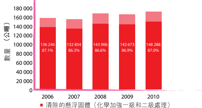
2006年至2010年在 污水處理過程中清除的懸浮固體
